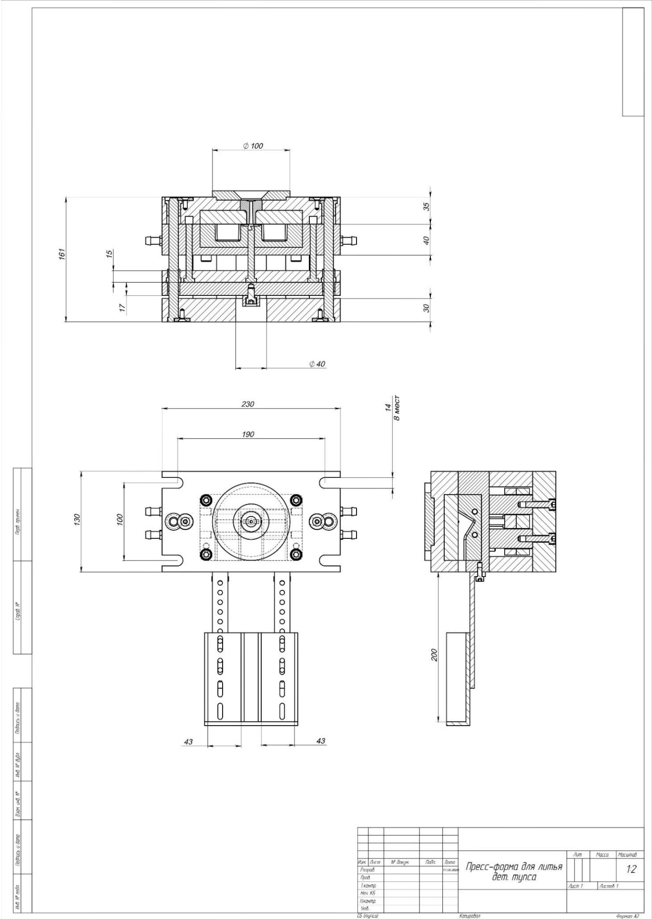
Рис.1 Чертеж пресс-формы для литья тупсы;
